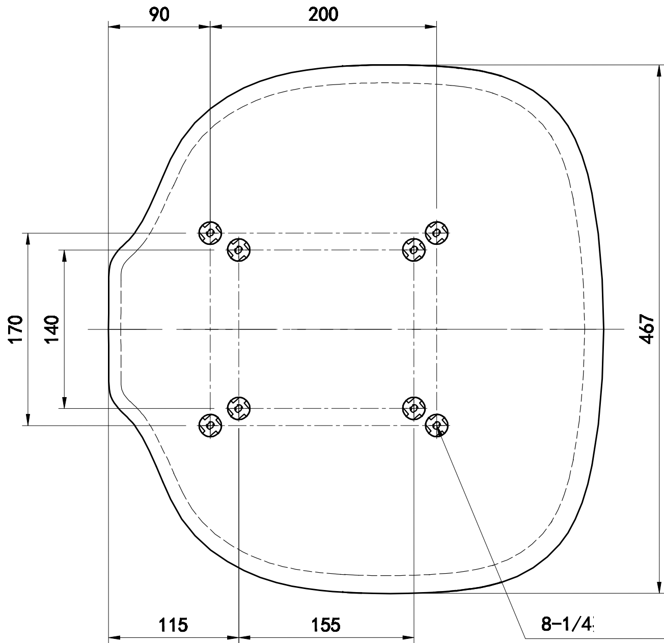
SDU-049 BLK PU Seat
