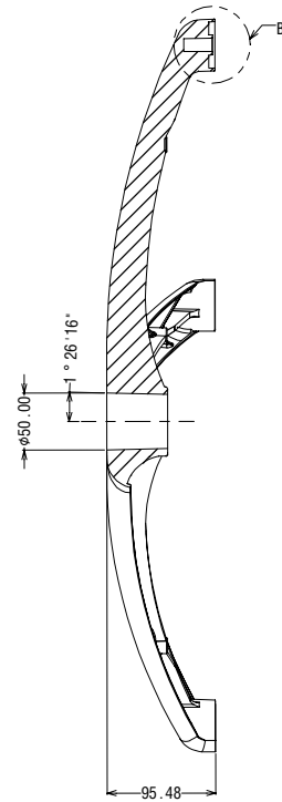
SECTION A-A
